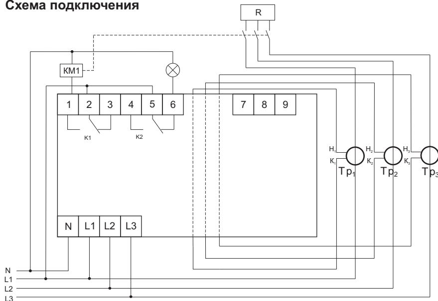
Рис.1 Схема включения с контактором и выходом для сигнализации о перегрузке по мощности.
