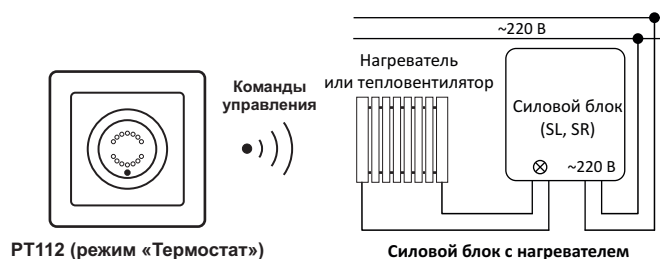
Рисунок 3. Использование датчика в качестве термостата
